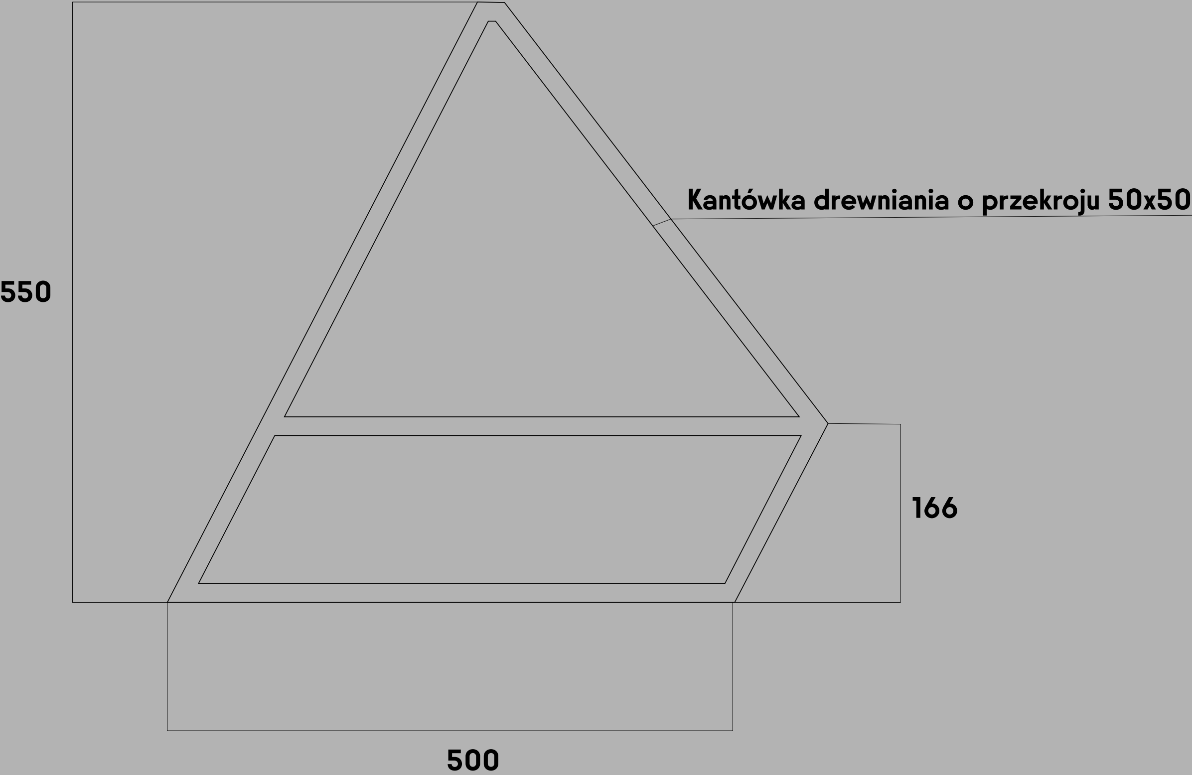
Rzut Góry
